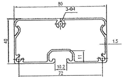
2.2. Conduit X-Section : 40 x 80 Heavy
