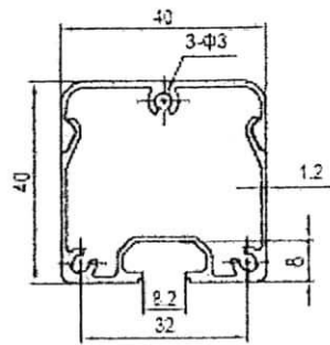
Conduit Profile-40x40 线槽型材-40x40
