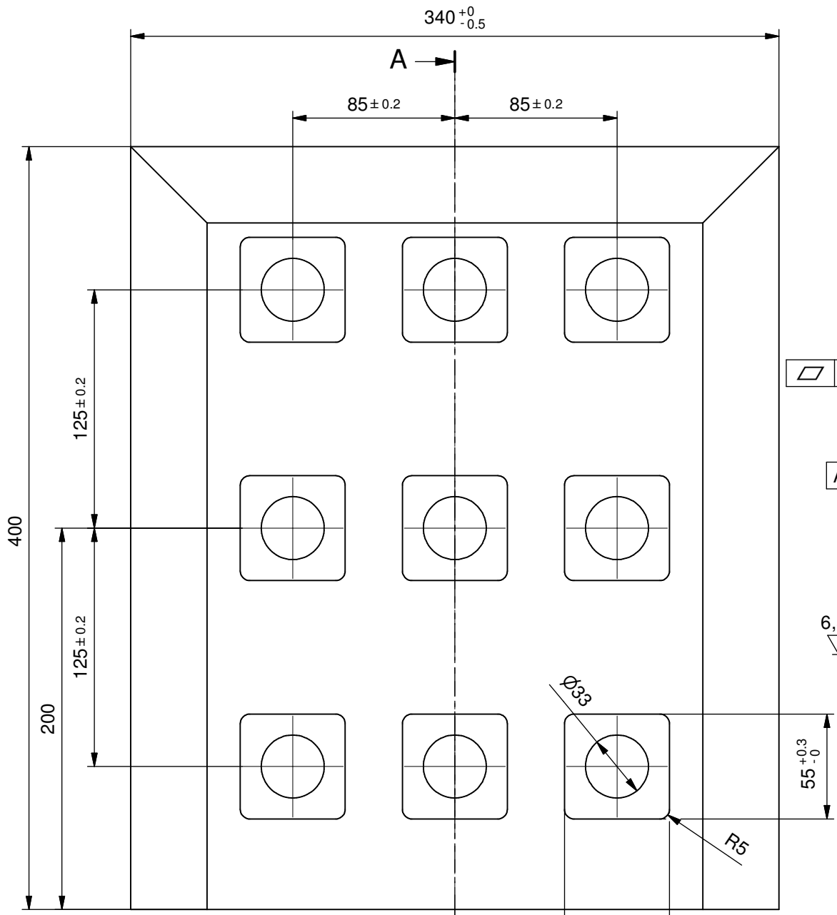
Item 1 (1:2)
