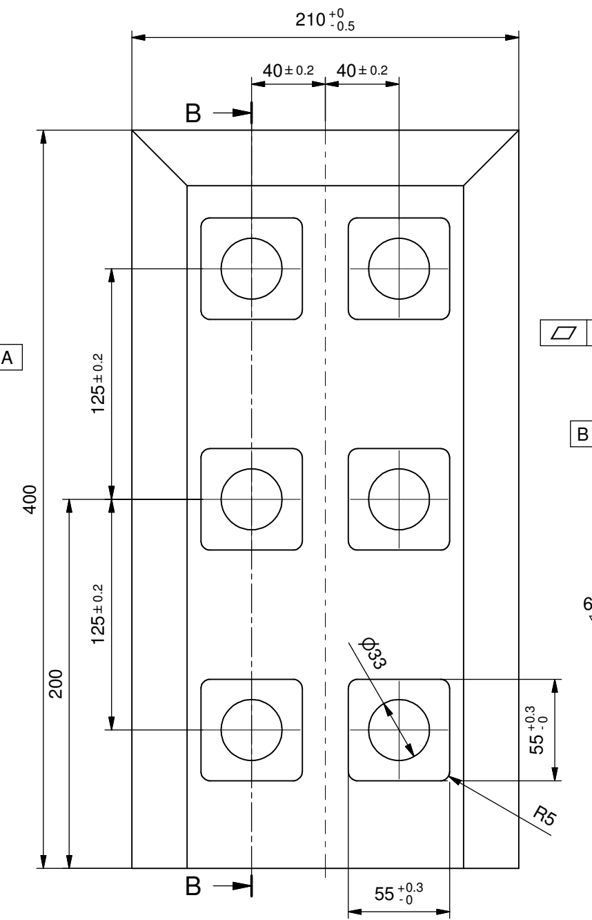
Item 2 (1:2)
