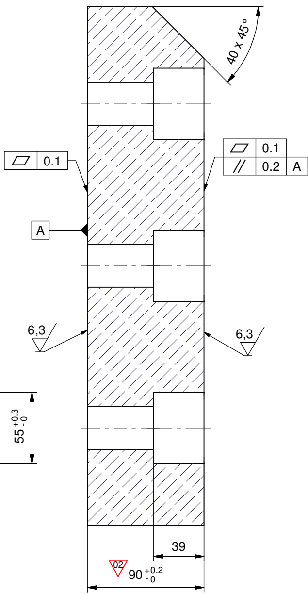
A-A (1:2)
