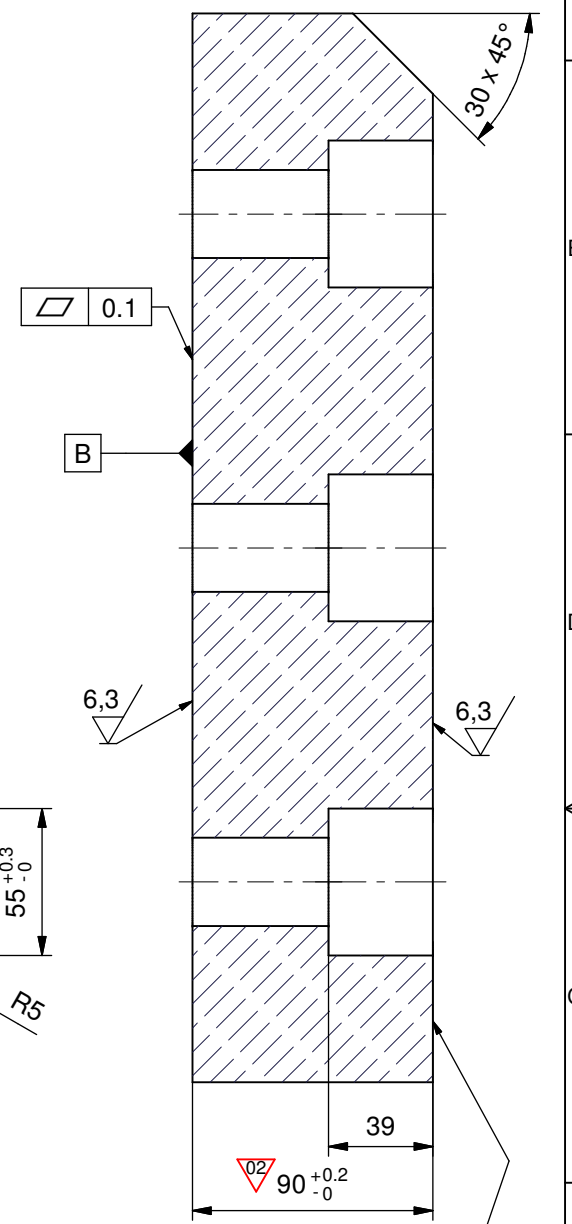
B-B (1:2)
